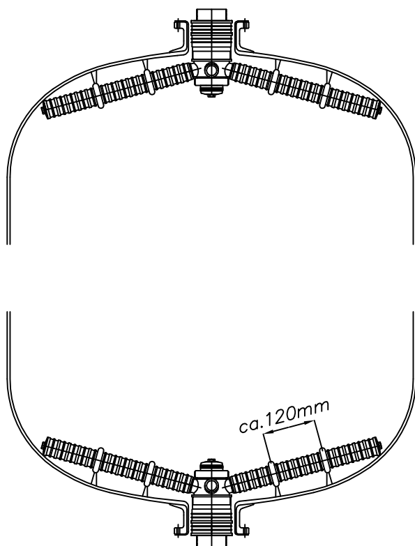
Abstützungen Supports
